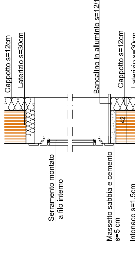
PARTICOLARE D-D scala 1:20
